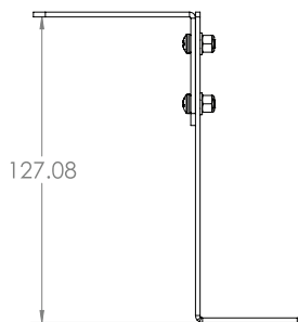
MAX HEIGHT
